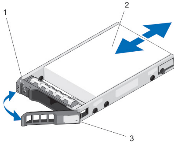
그림 20. 핫 스왑 하드 드라이브 분리 및 설치
