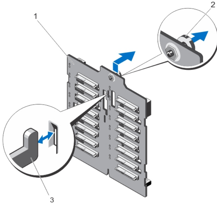
그림 31 . x16 하드 드라이브 후면판 분리 및 설치
