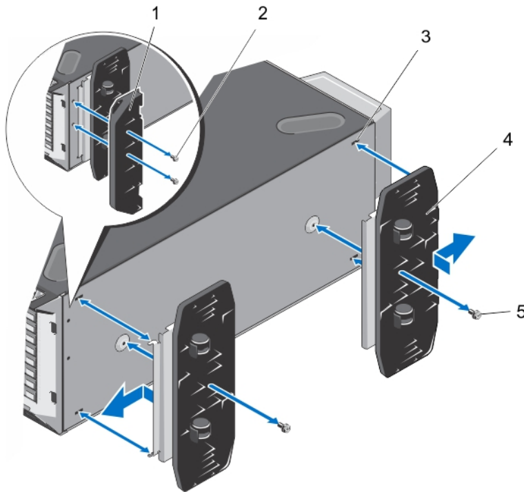
그림 13. 휠 조립품 분리 및 설치
