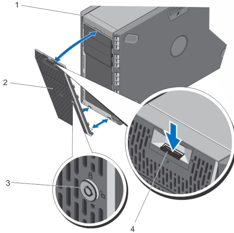
그림 11. 전면 베젤 분리 및 설치
