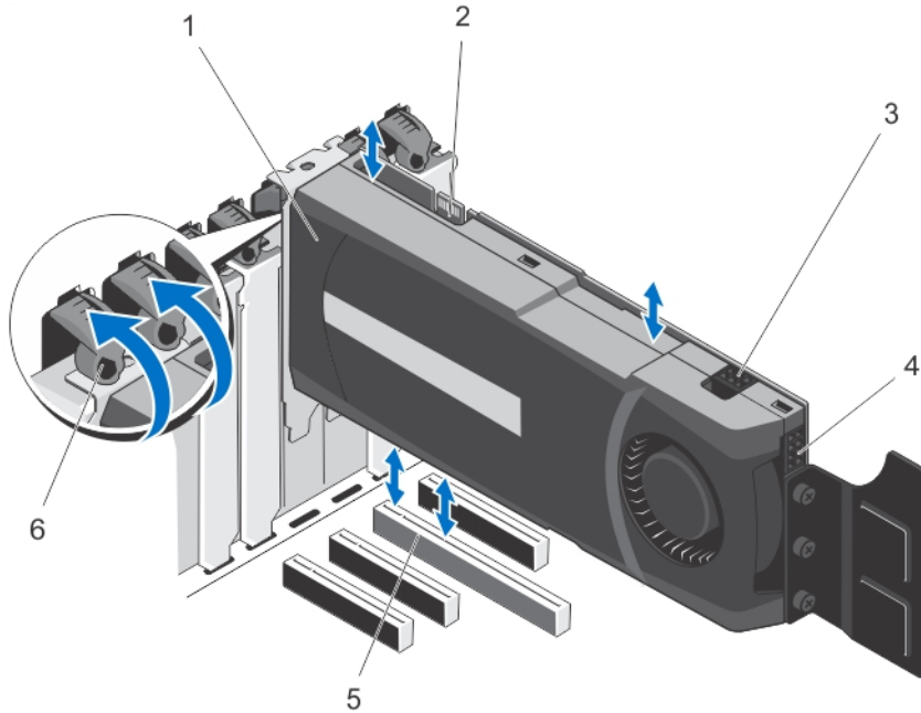
그림 46. GPU 카드 분리 및 설치
