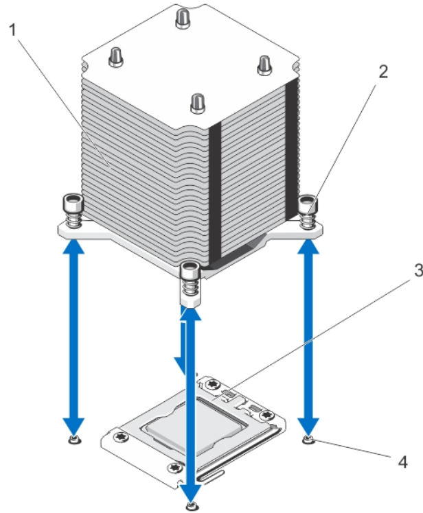
그림 50. 방열판 분리 및 설치
