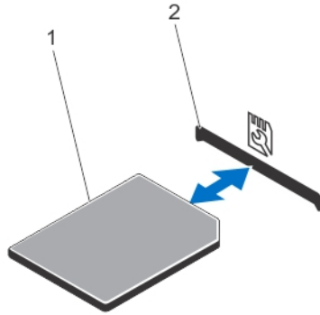
그림 48. SD vFlash 카드 분리 및 설치
