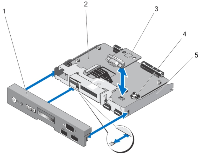
그림 67. VGA 모듈 분리 및 설치
