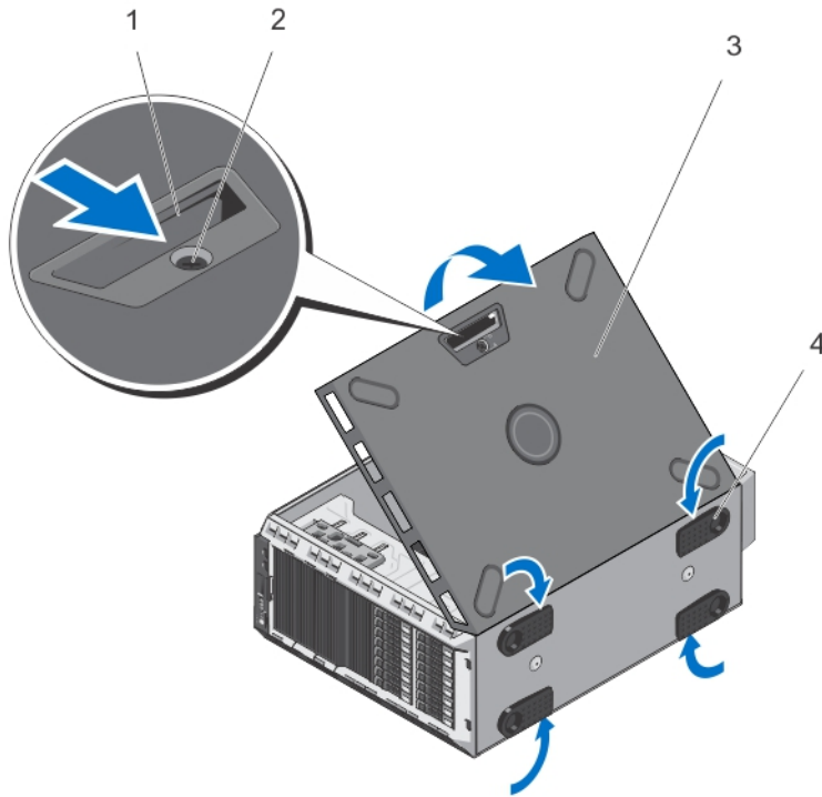
그림 14. 시스템 열기 및 닫기
