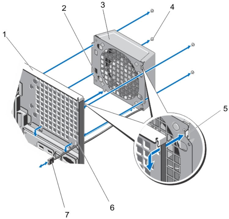
그림 41. 외부 냉각팬 분리 및 설치
