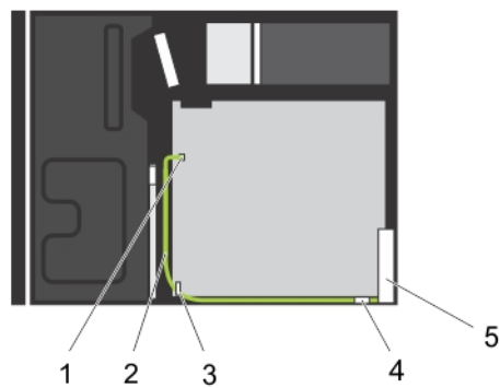
그림 40. 케이블 연결—내부 냉각 팬
