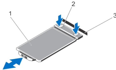
그림 61. 정보 태그 분리 및 설치
