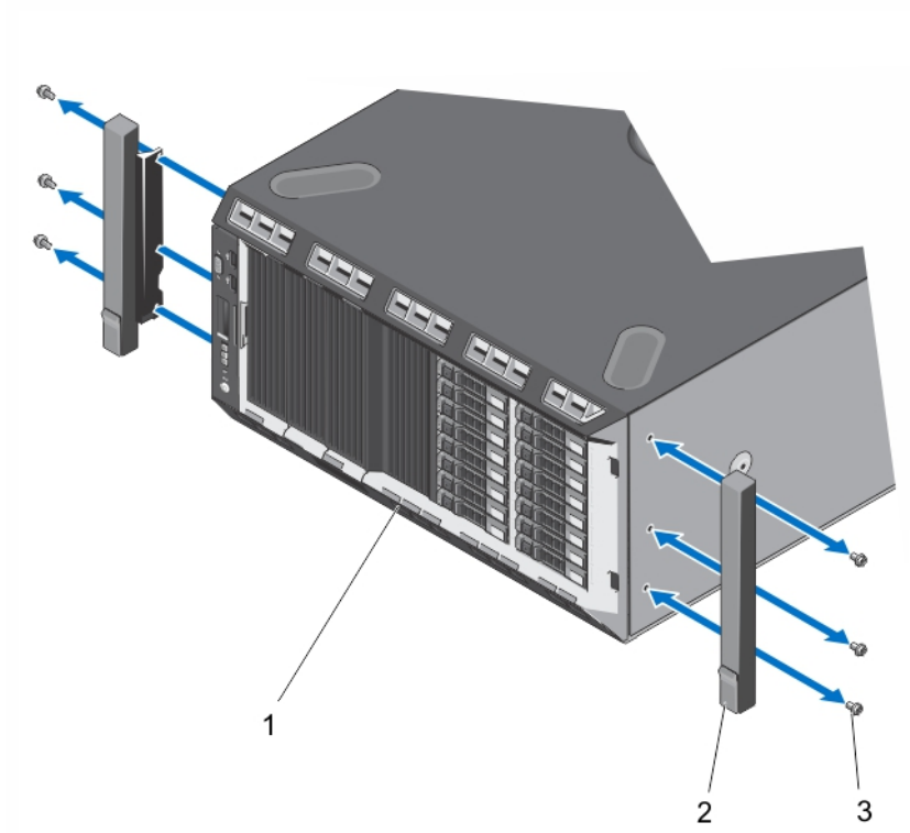
그림 70. 랙 이어 분리 및 설치
