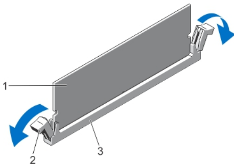
그림 36. 메모리 모듈 배출
