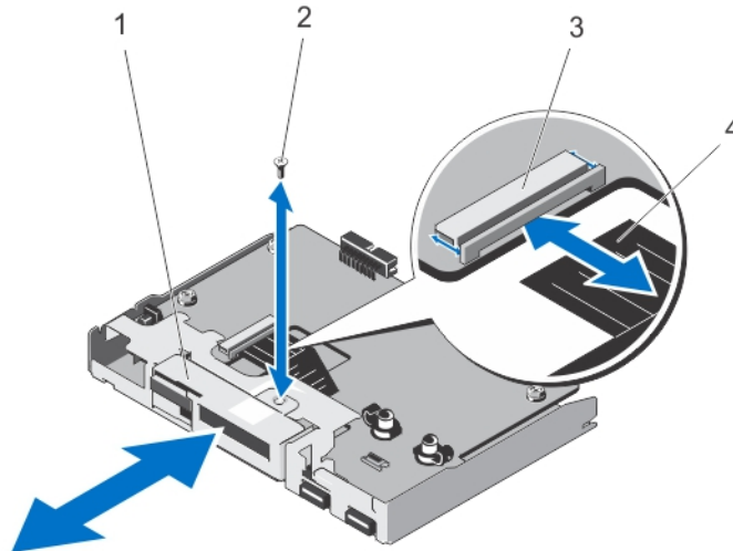
그림 66. LCD 모듈 분리 및 설치
