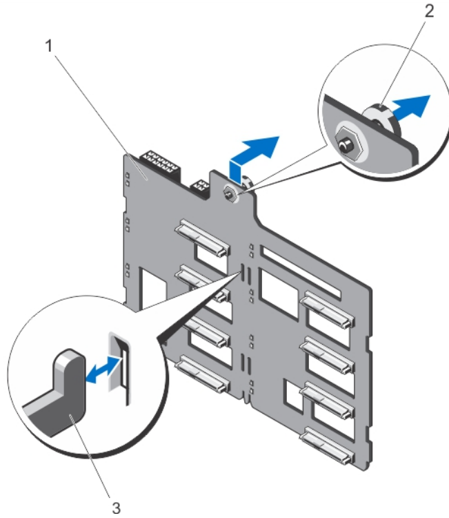
그림 28. x8 하드 드라이브 후면판 분리 및 설치
