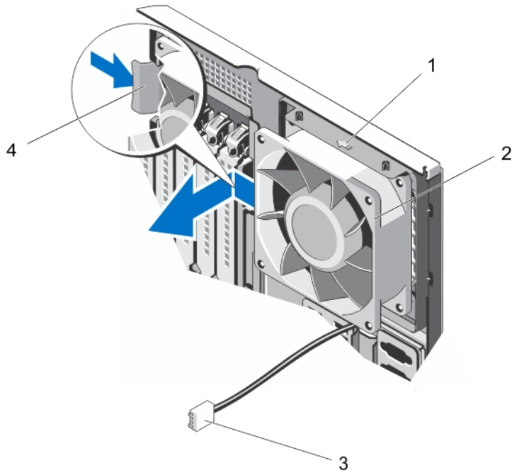
그림 39. 내부 냉각팬 분리 및 설치
