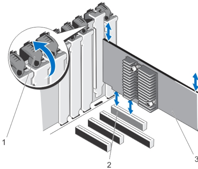
그림 45. 확장 카드 분리 및 설치
