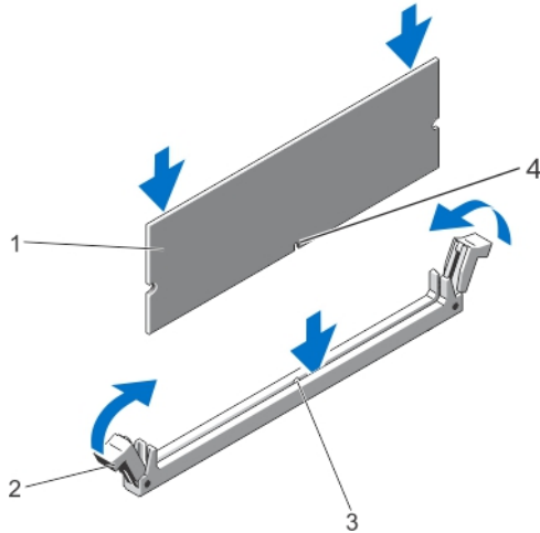
그림 38. 메모리 모듈 장착
