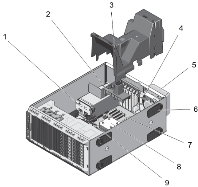
그림 15. 시스템 내부—핫 스왑 가능한 하드 드라이브
