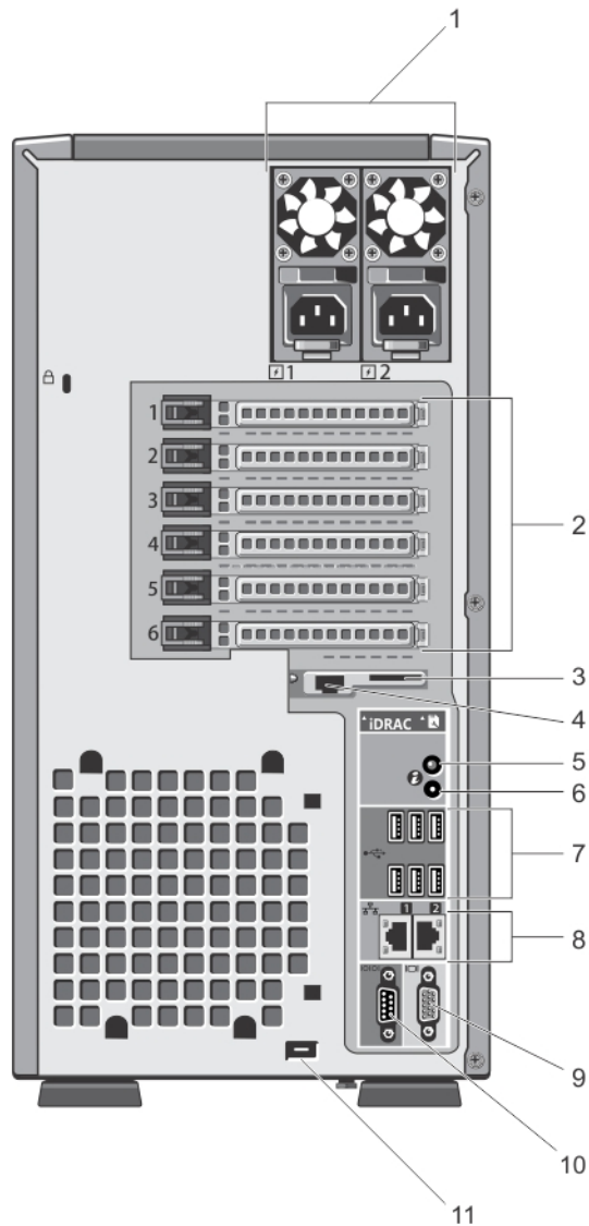
그림 7. 후면 패널 구조 및 표시등
