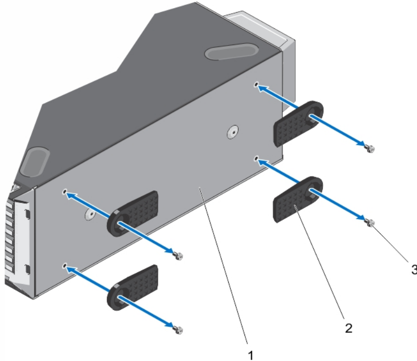
그림 12. 시스템 다리 분리 및 설치
