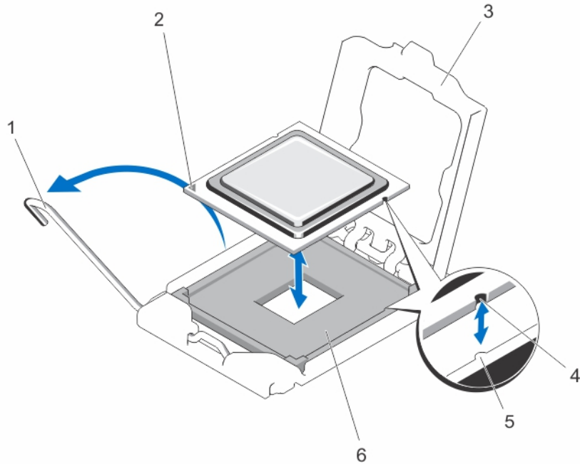
그림 51. 프로세서 분리 및 설치
