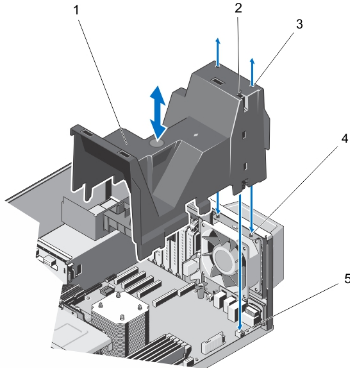
그림 19. 냉각 덮개 분리 및 설치
