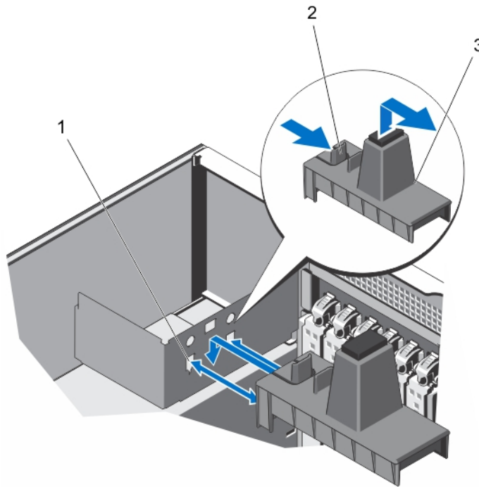
그림 44. PCIe 카드 홀더 분리 및 설치
