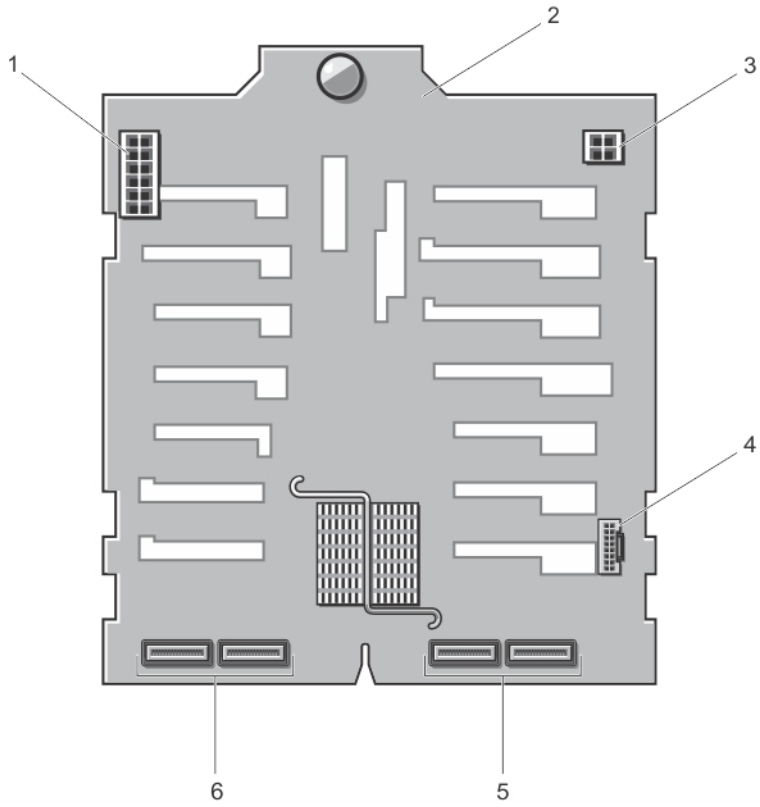
그림 32. x16 하드 드라이브 후면판의 커넥터
